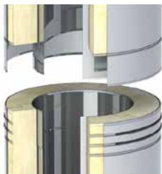
Sistema de unión Macho-Hembra, cónico interior con abrazadera 2.0 exterior.
